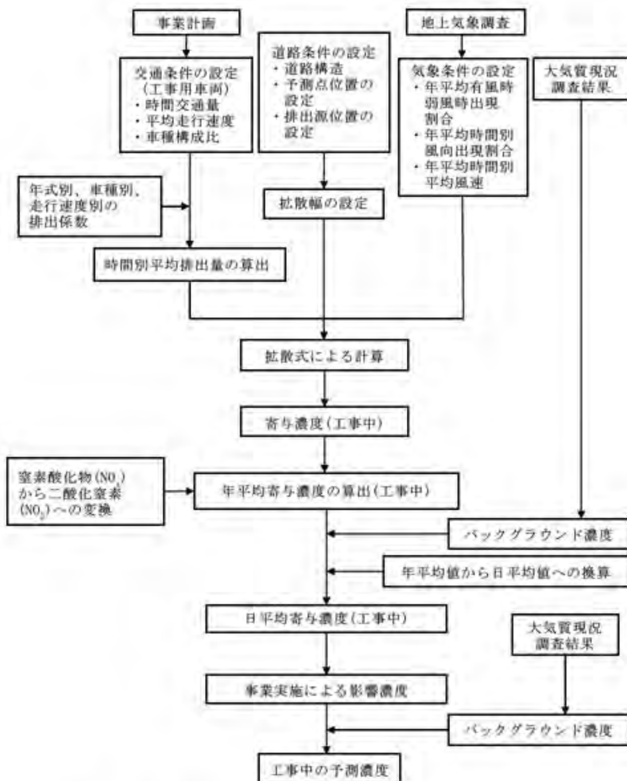
図 6.1-14 資材等の運搬車両の走行に伴う排出ガスの予測手順
