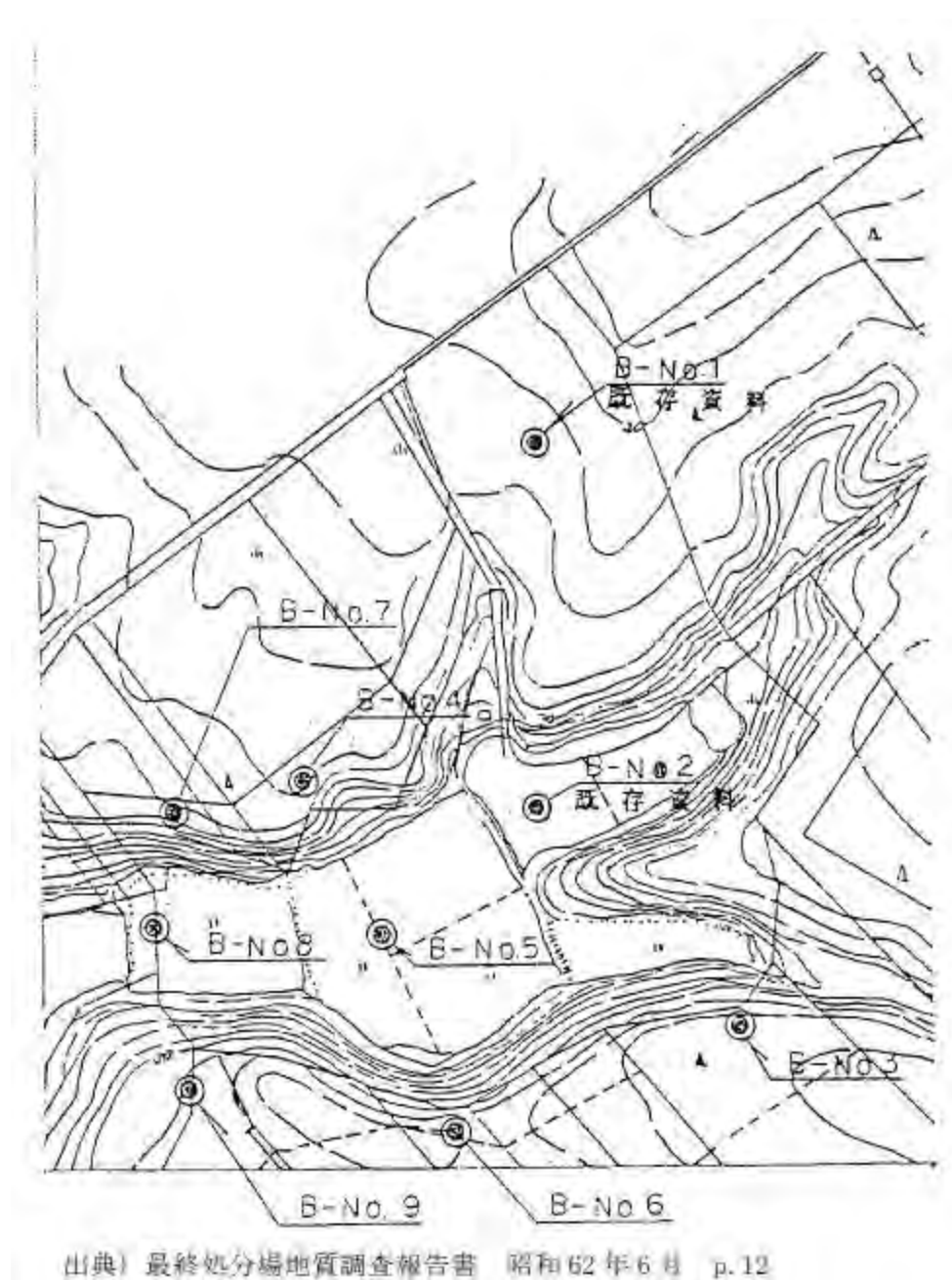
図 6.9-2 対象事業地の地質調査位置図
