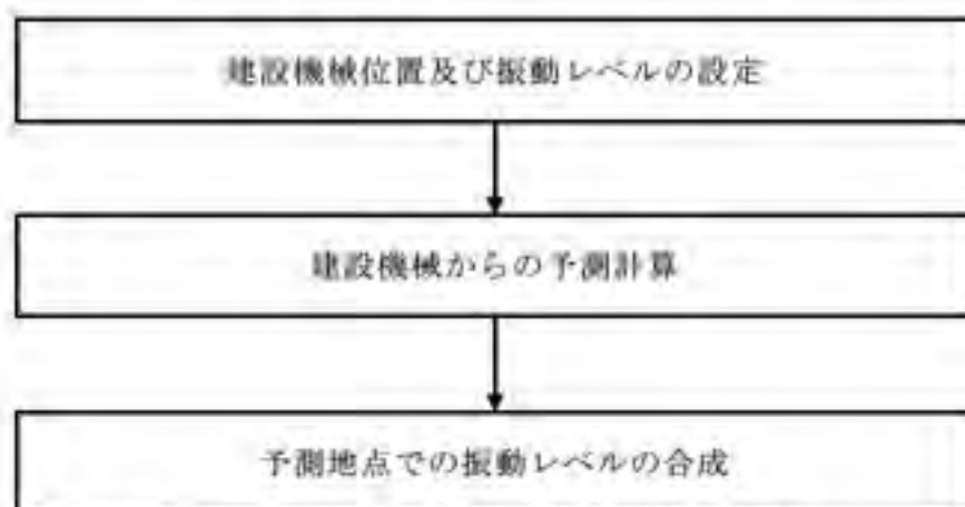
図 6.3-3 施設稼働による振動の予測手順
