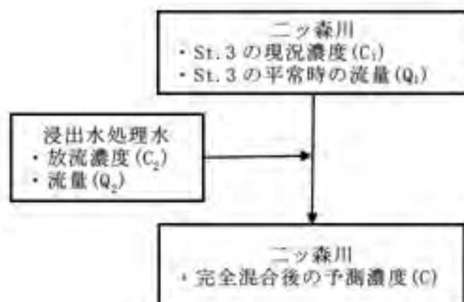
図 6.5-7 予測モデル(浸出水処理水による水質)
