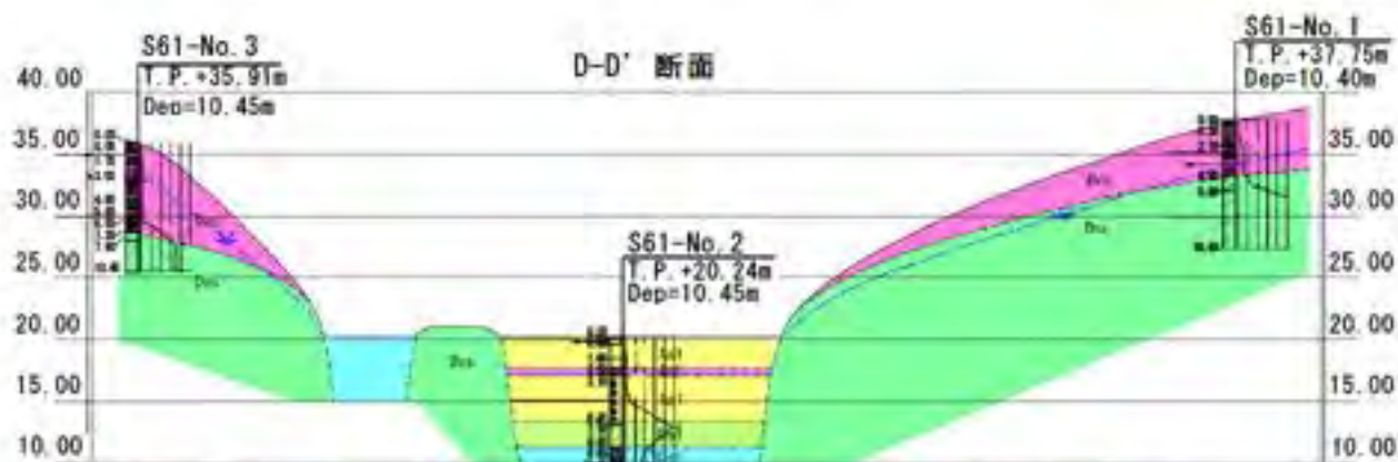
図 6.7-4 断面 1：造成に伴う土地改変と地下水との関係（上流部）
