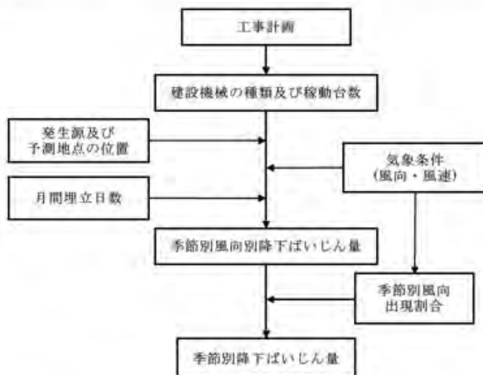
図 6.1-22 建設作業機械の稼働に伴う粉じん(降下ばいじん)の影響の予測手順
