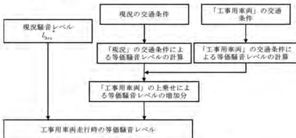
図 6.2-2 資材等の運搬車両の走行に伴う騒音の予測手順
