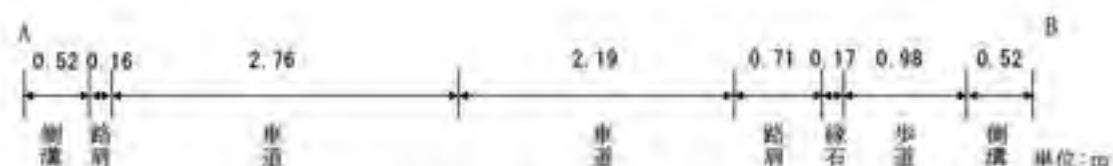
図 6.1-13 国道の道路構造 (St. 3 : 南側沿道地点)
