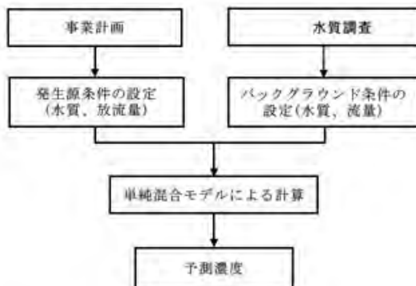
図 6.5-4 造成等の施工による水の濁りの影響の予測手順
