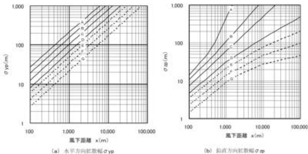
図 6.1-19 風下距離の関数としての Pasquill-Gifford の \sigma_{yp} 、 \sigma_{zp}
