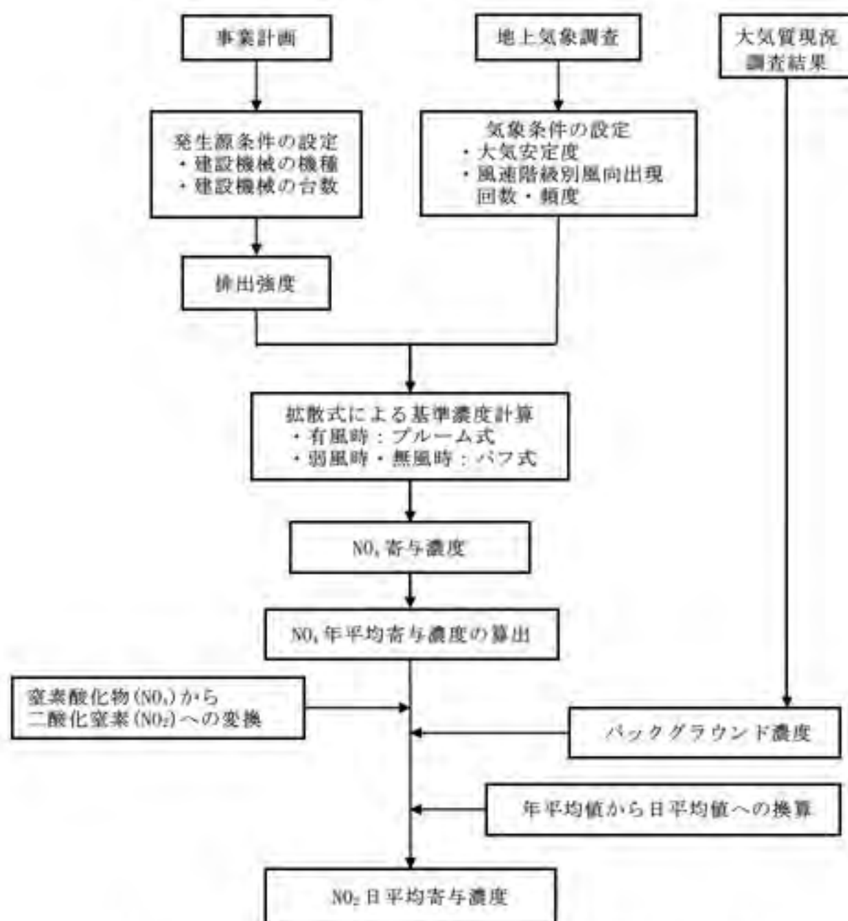
図 6.1-18 建設作業機械の稼働に伴う排出ガスによる影響の予測手順
