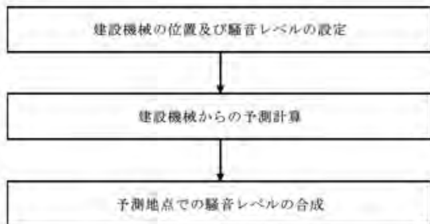
図 6.2-4 建設機械騒音の予測手順
