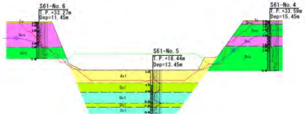
図 6.9-6 AA' 断面：造成に伴う土地改変と地下水との関係(中流部)
