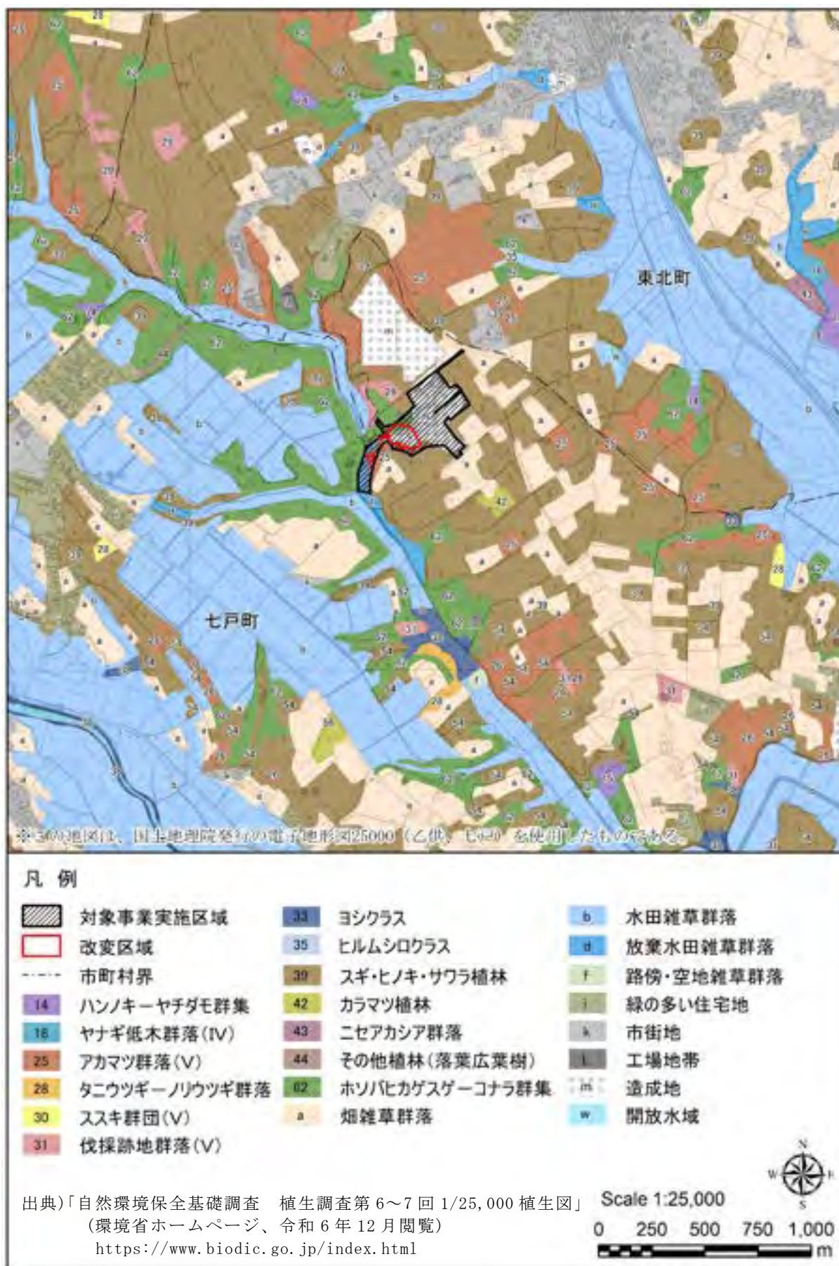
図 3.1-14 現存植生図
