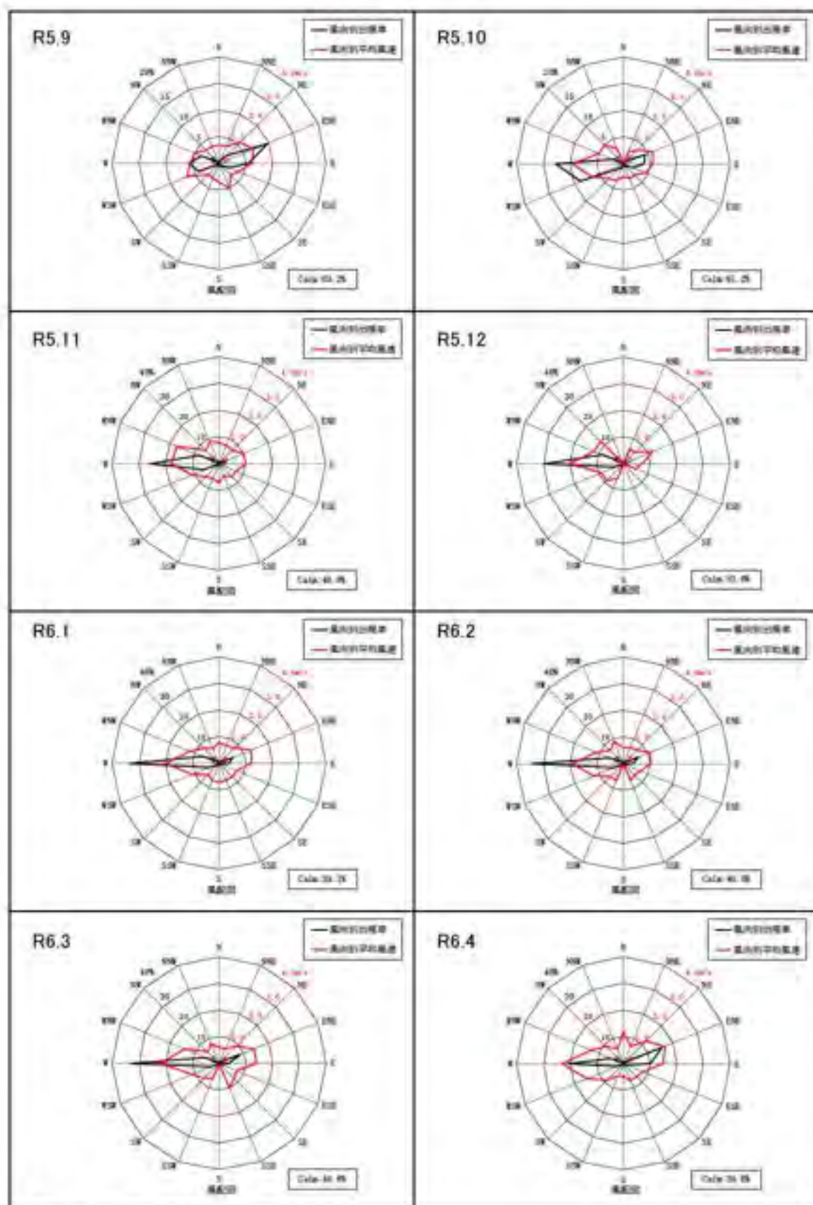
図 6.1-7(1) 月別風配図
